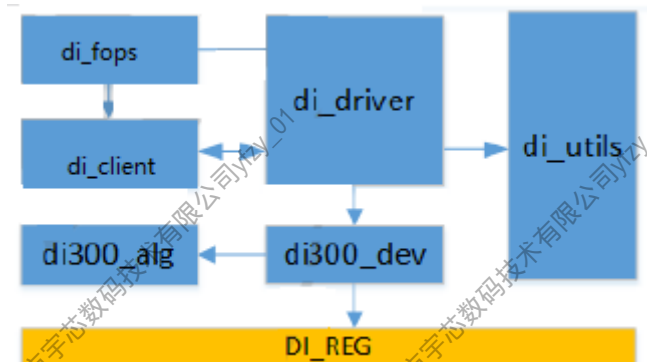
图 2-4: DI 驱动结构
