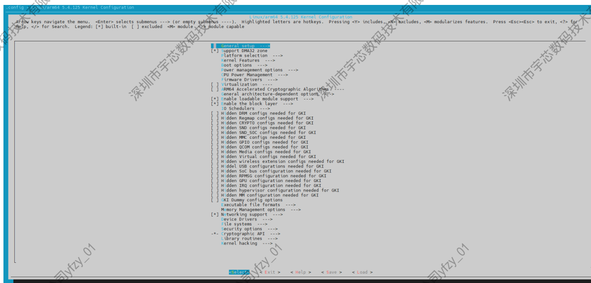
图 2-2: menuconfig 主界面
