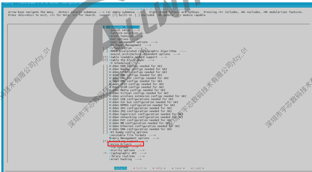
图 2-5: menuconfig 主界面
