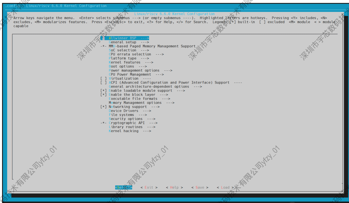
图 2-6: menuconfig 根目录
