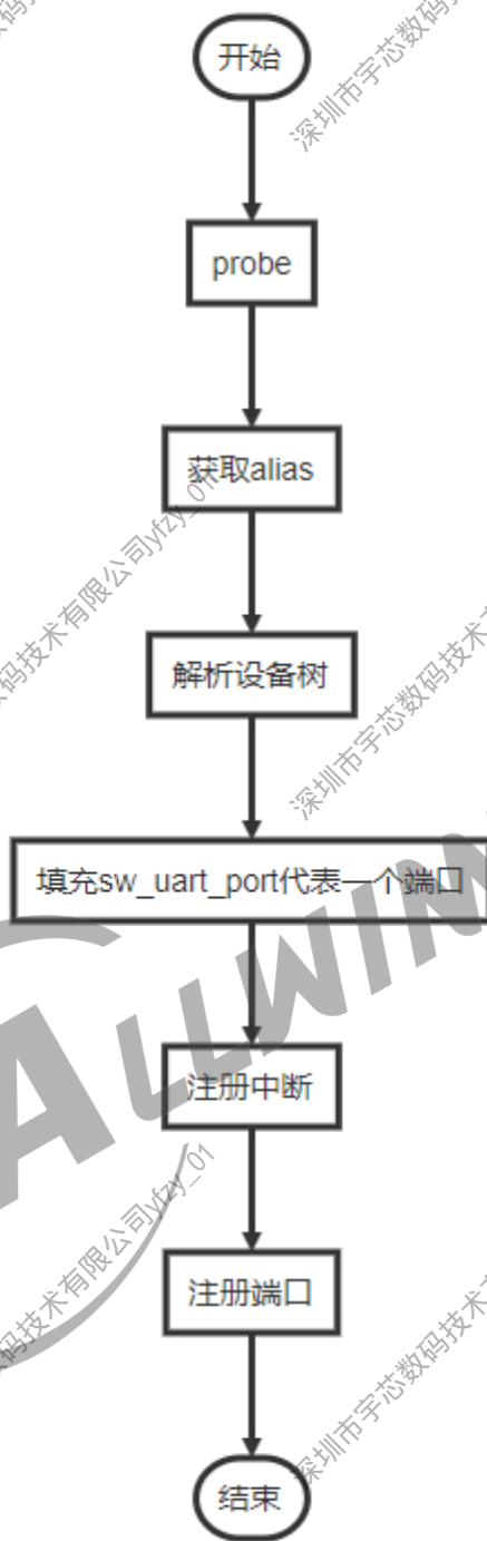
图 2-1: 初始化流程
