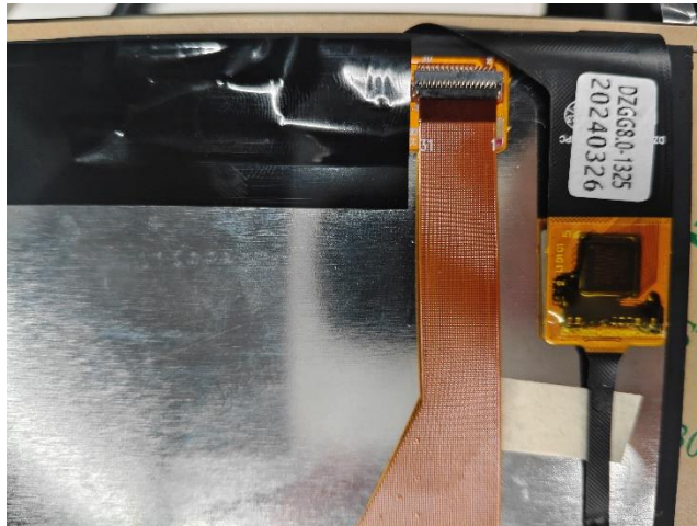
(7) mipi8_800x1280 屏幕背面连接图
