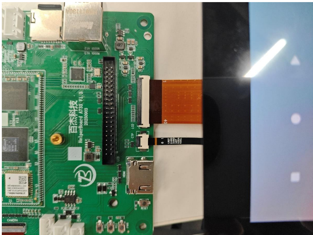
(6) mipi8_800x1280 屏幕连接图
