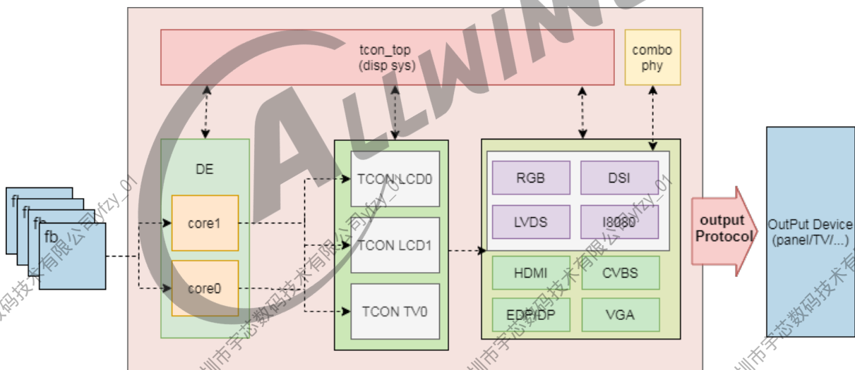
图 2-3: 硬件概览
