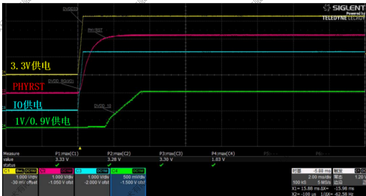
图 6-8: 上电时序
