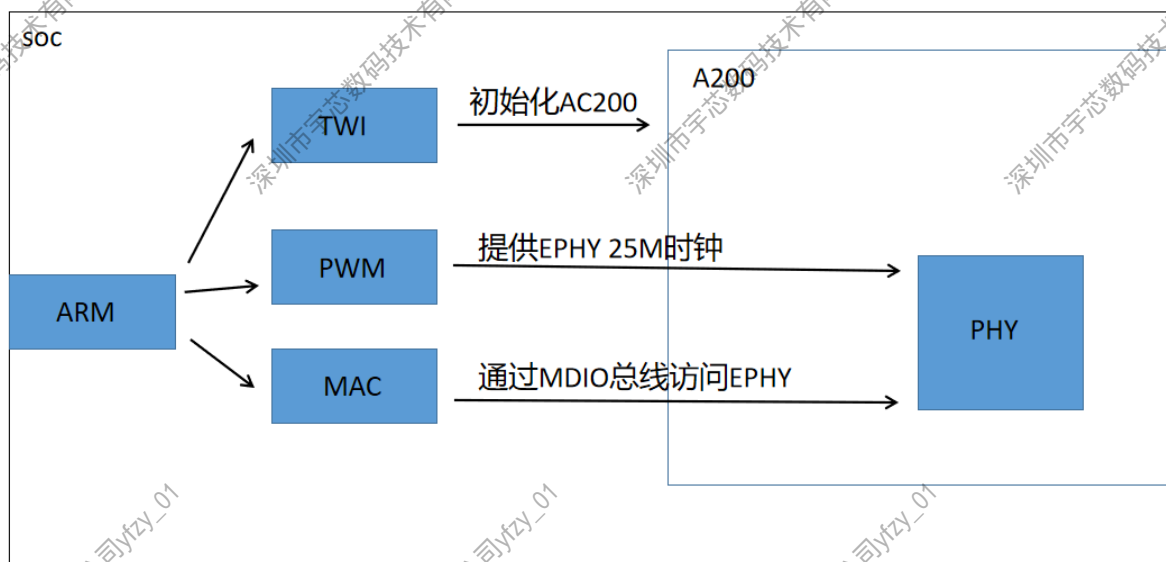
图 3-3: AC200 框图
