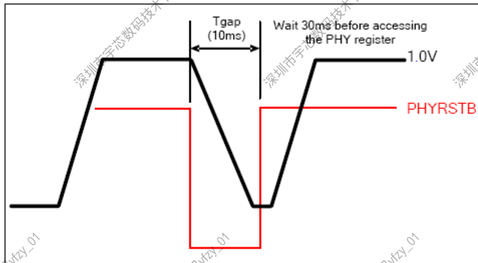
图 6-9: 复位时序
