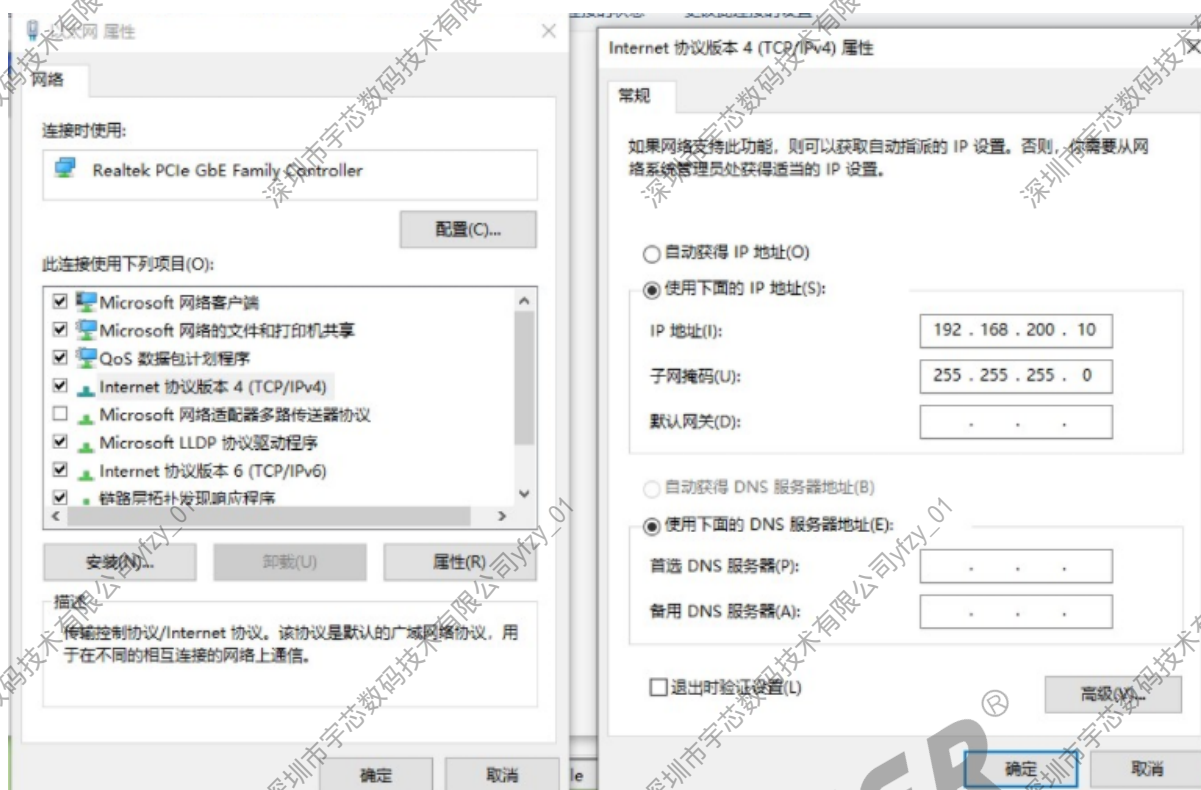
图 7-6: 配置 IP
