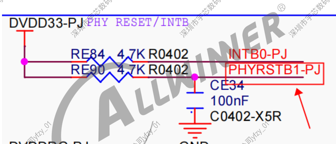
图 6-10: phyrst 原理图
