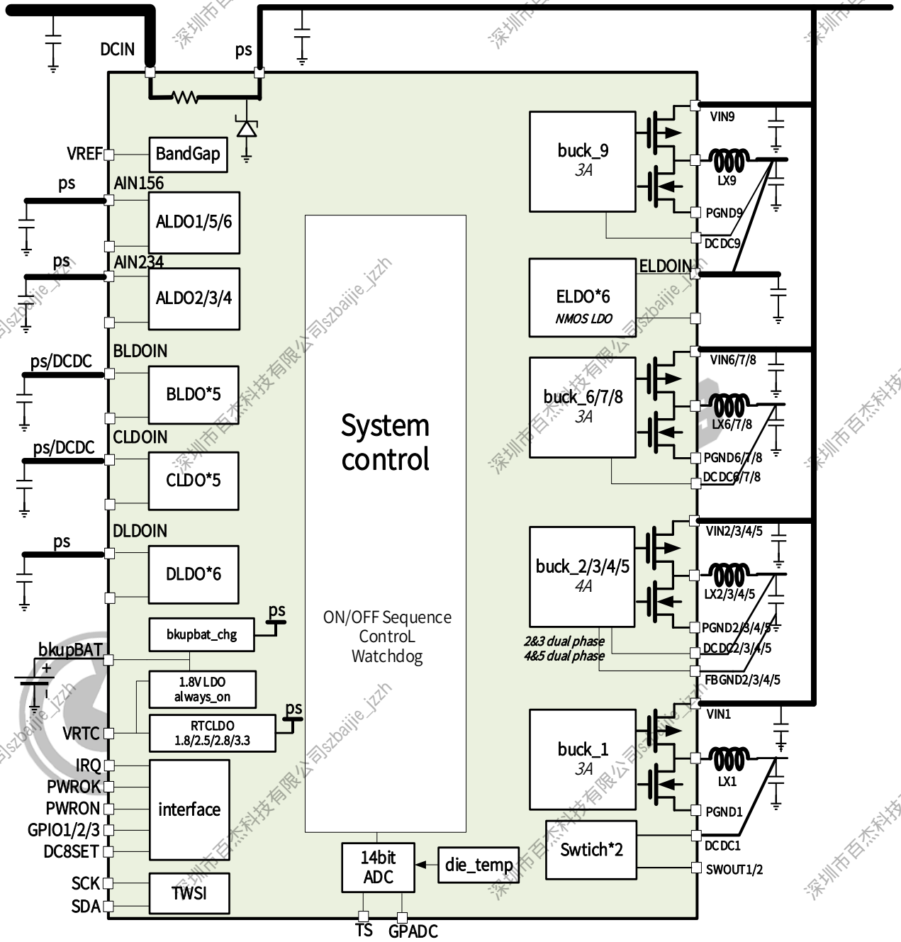
图 6-1 结构框图
