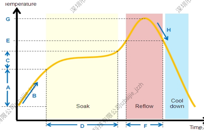
图 10-1 典型回流焊曲线
