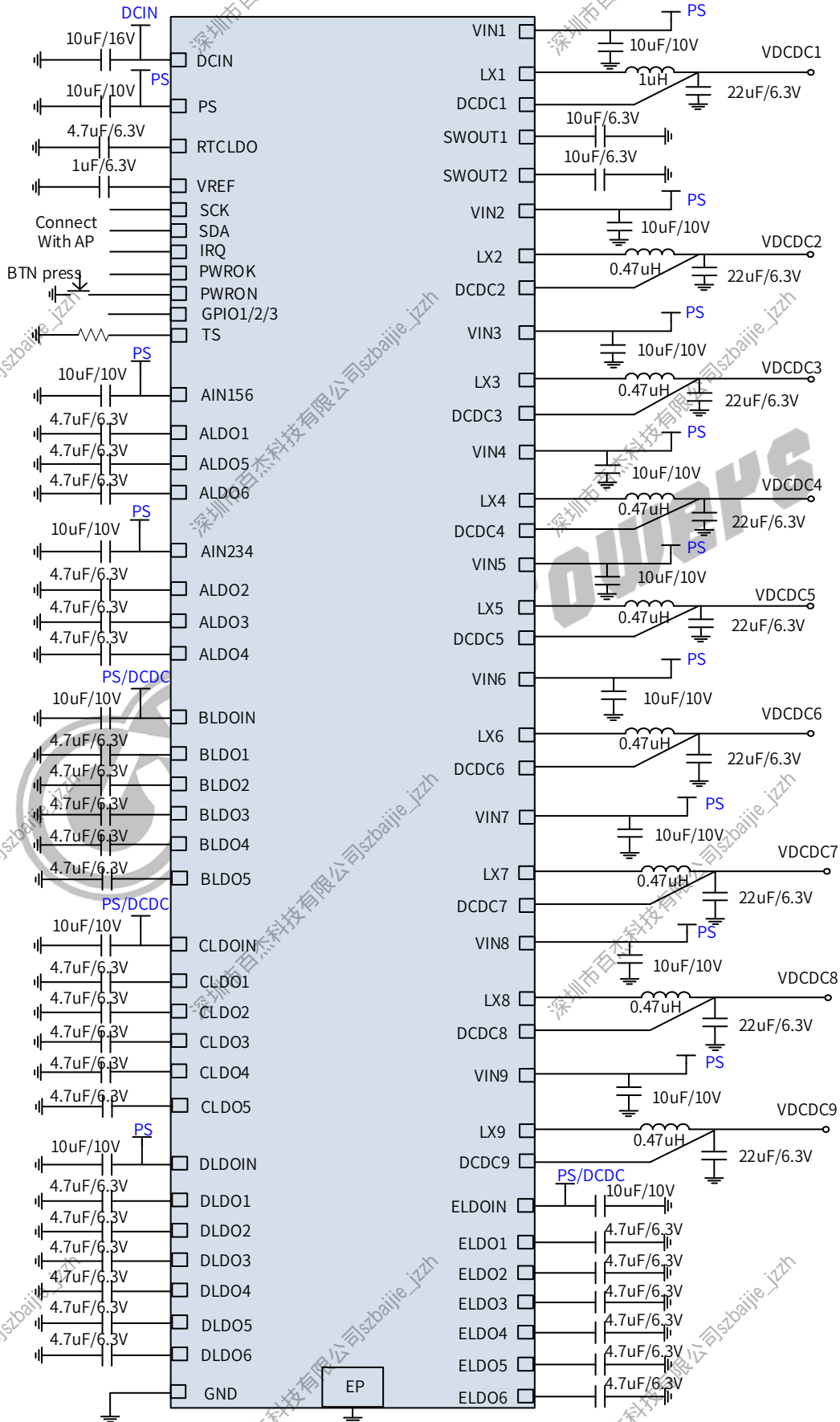
图 7-1 典型应用图
