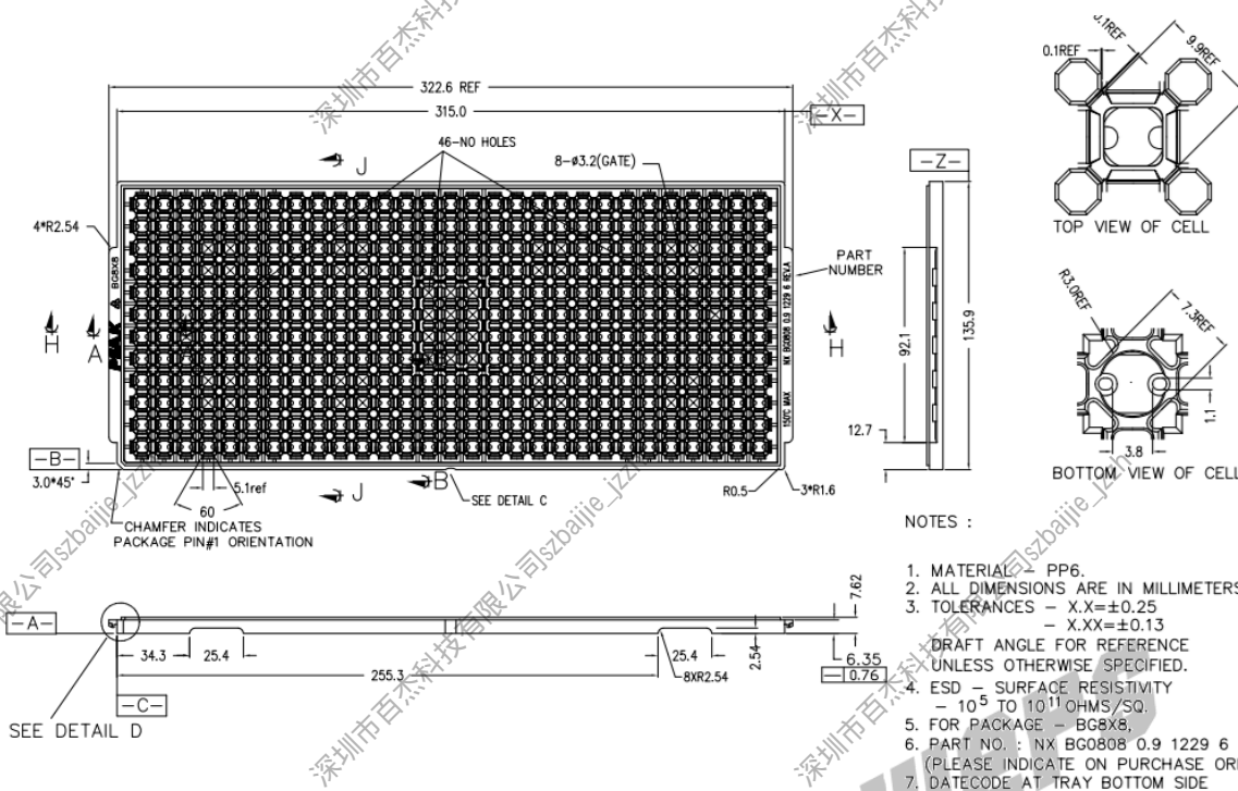
图 9-3 托盘尺寸图
