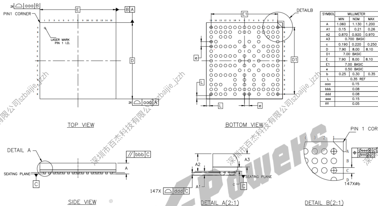
图 9-2 丝印图
